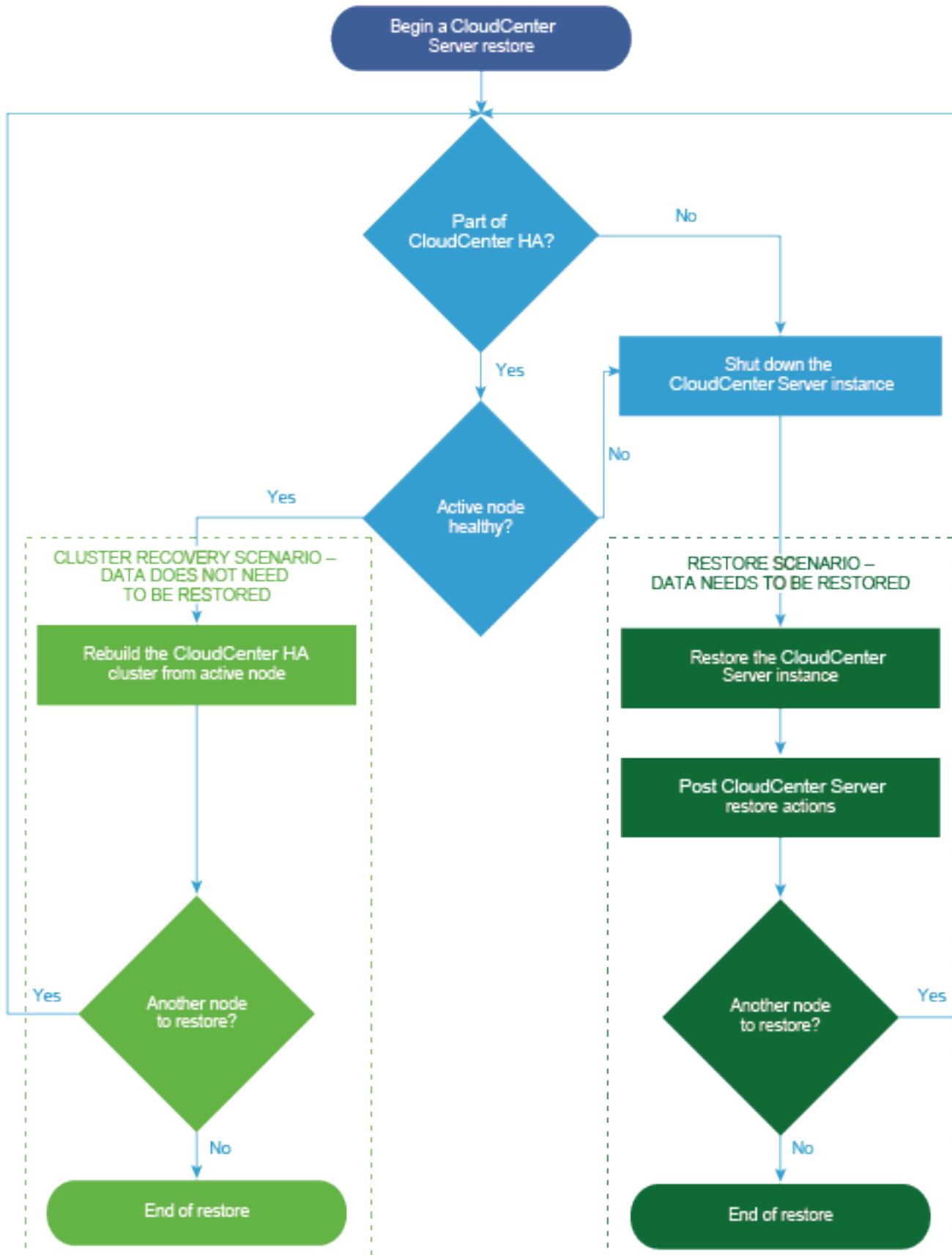
图 7-1 vCenter Server 还原 workflow
