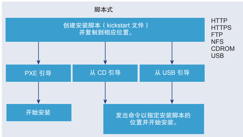
图 2-1 脚本式安装
