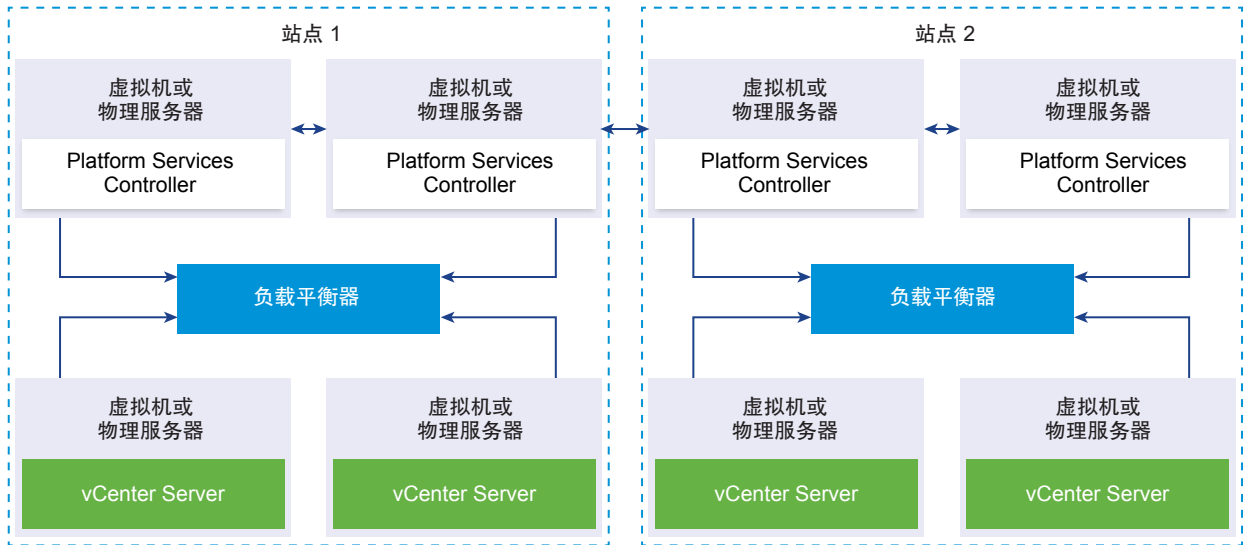
图 1-7 跨两个站点并实现了负载均衡的两个 Platform Services Controller 实例对的示例
