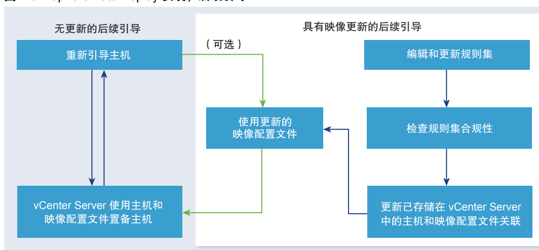
图 2-6 vSphere Auto Deploy 安装，后续引导
