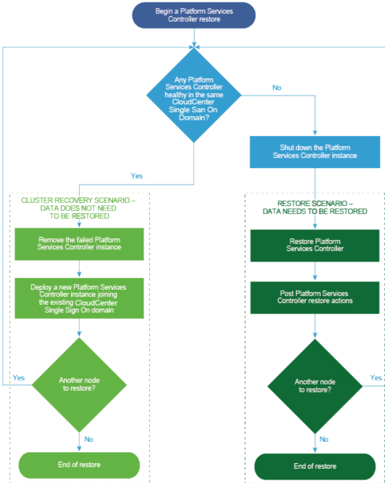
图 6-2 Platform Services Controller 设备还原 workflow
