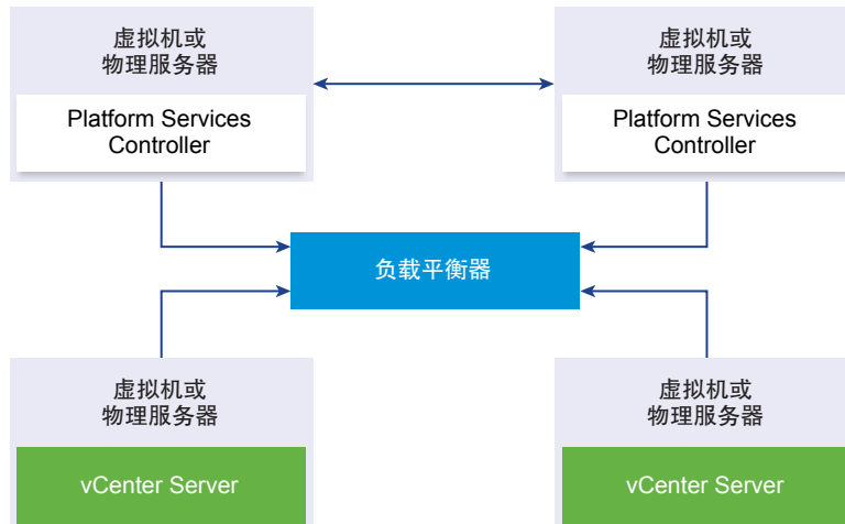
图 1-6 实现了负载平衡的 Platform Services Controller 实例对的示例
