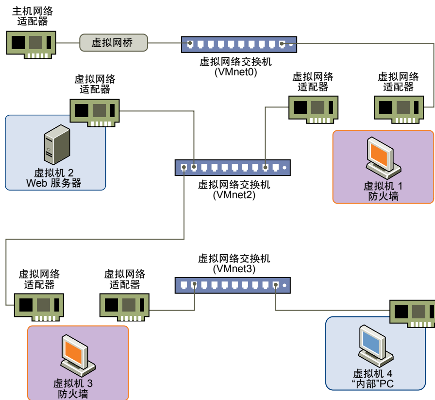
图 9-4 具有两个防火墙的自定义配置
