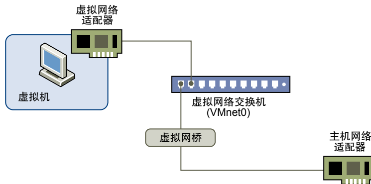
图 9-1 桥接模式网络连接配置
