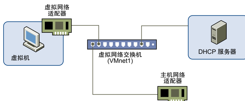
图 9-3 仅主机模式网络连接配置
