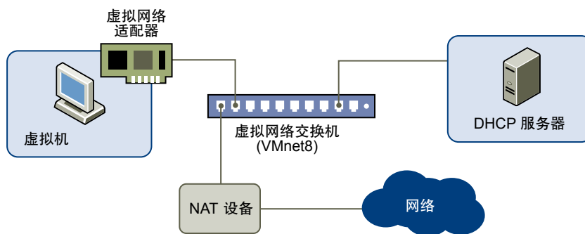
图 9-2 NAT 配置
