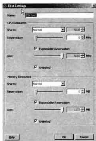
▲ 内存和 CPU 的分配是资源池的最重要任务
