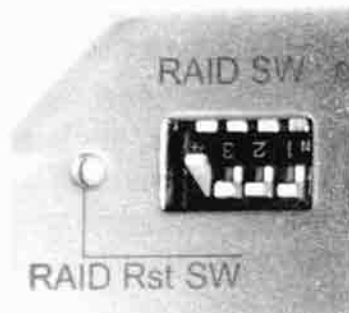
▲ 这是使用 Switch 配置 RAID 的 NAS
