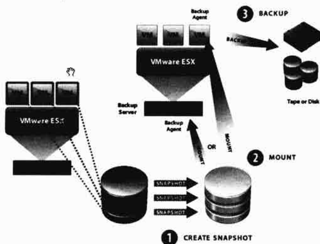
▲ VCB 的架构图
