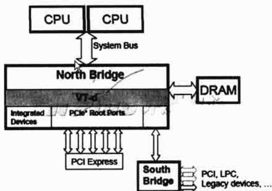
▲ 这是标准的直接硬件访问示意图
