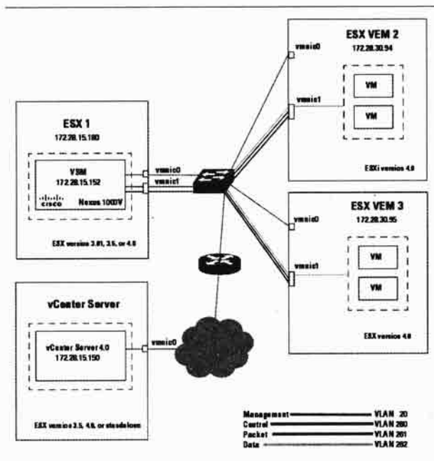
▲ Nexus 1000V 架构图 (取自 Cisco 网站)
