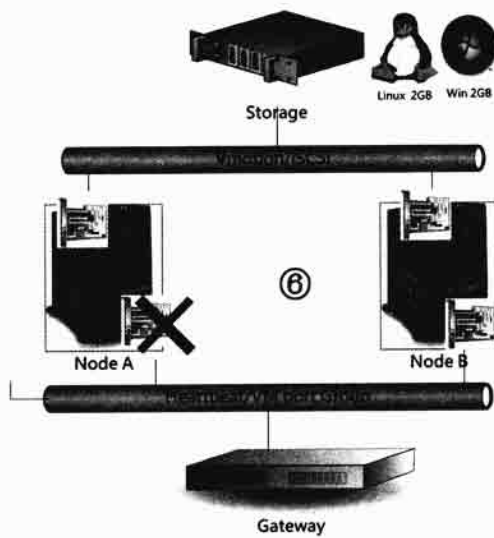
▲ 计算机 A 发现自身坏了，就去存储设备解锁虚拟机准备释出
