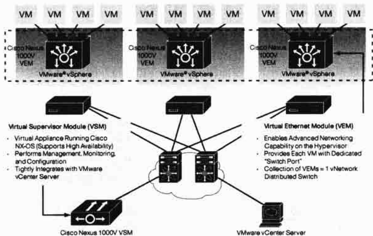
▲ 图为 VN-LINK 的架构（取自 Cisco 网站）
