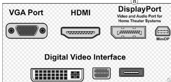
⑧ • DP接口和其他接口的外观差异
