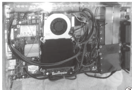
⑦ • 平板机箱内实物图
