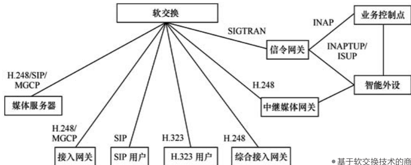
• 基于软交换技术的商用组网方式
