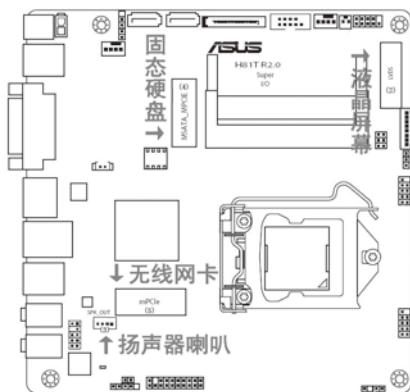
③ 文中第(2)(3)(4)条所提到的接口，详见本图中各文字标记处
