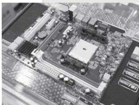
> 杰微JWA75VM主板实际采用的是AMD A55芯片
