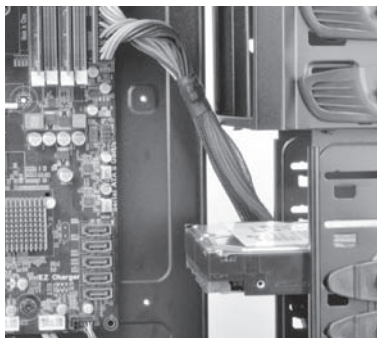
24PIN电源走线
