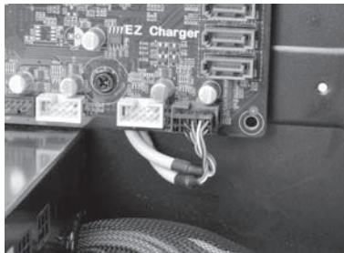
前置USB引线从主板底部穿过来
