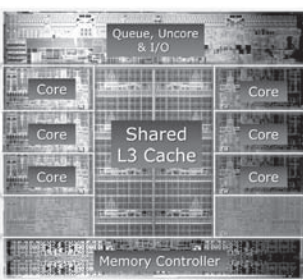
六核心分布示意图
