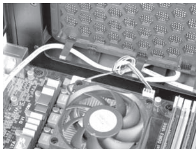
前置音频线可以通过边缘走到主板的安装位
