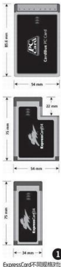
ExpressCard不同规格对比
