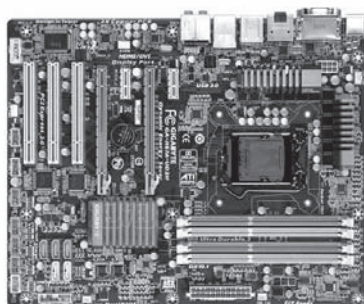
ATX规格的技嘉GA-H67A-UD3H主板
