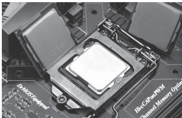
▲LGA1155取代LGA1156,还好老散热器依然可用
