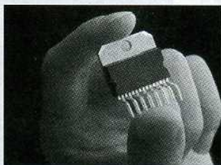
▲低音单元采用的TDA7296是意法半导体生产的一颗HIFI级的单声道大功率功放芯片,能提供60W的输出功率,这比很多2.1音箱的低音通道所用的“大功率功放”功率还要大得多
