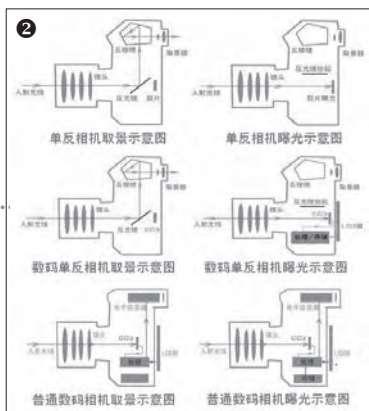
▲传统单反、数码单反、普通数码相机原理对比
