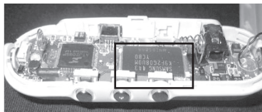
▲MP3中的三星闪存芯片
