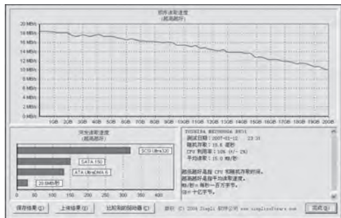
让人感到惊异的是这款移动硬盘竟然拥有如此快速的传输速度,十分优秀,而其体积不过比名片大些而已
