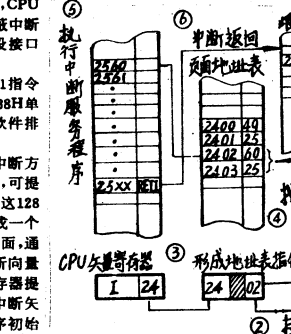
图2 方式2中断处理过程示意图
