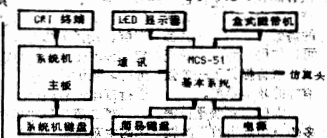
图 1 板级型 MCS-51 仿真器
