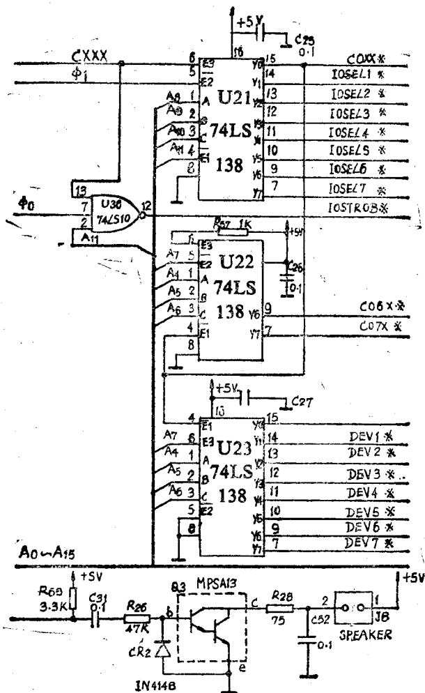
图9 I/O译码电路
