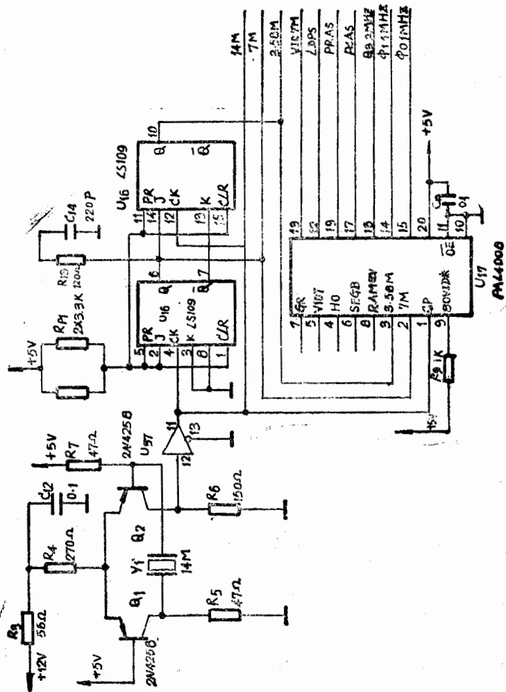
图 4 振荡器和系统时基电路
