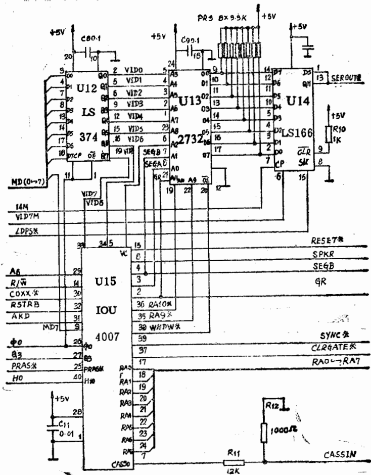
图 7 视频数据转换电路
