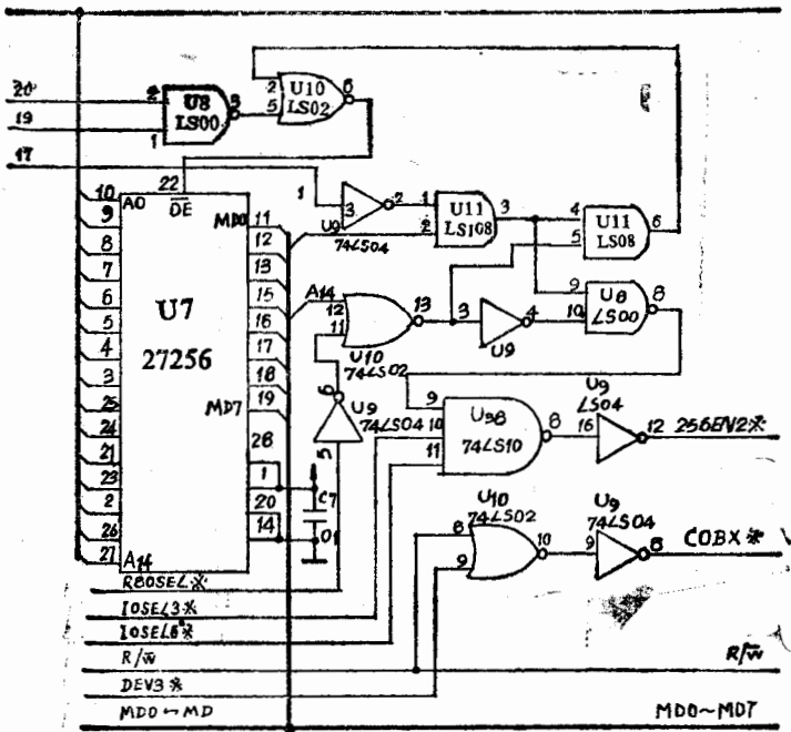
图6 存储器管理部件及相关电路(续)
