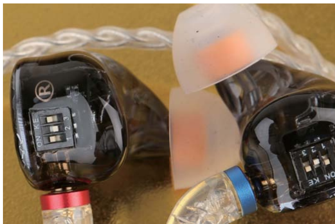
耳机的三档调音开关，控制高、中、低音以及高阻、低阻的调节与切换，用户通过它们可实现8种不同组合。
