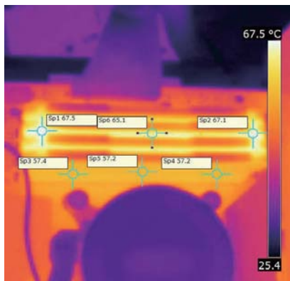
使用AIDA64对这套内存烤机半个小时之后，其最高温度为67.5°C，位于内存顶部，而散热马甲两侧的温度则控制在60°C以下。
