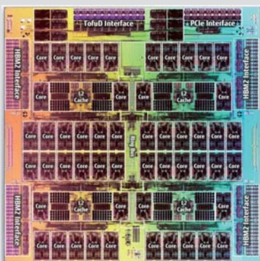
■ A64FX处理器内部布局图
