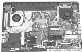
笔记本电脑散热系统是根据每一款产品的空间进行设计的，没有标准化的产品可更换
