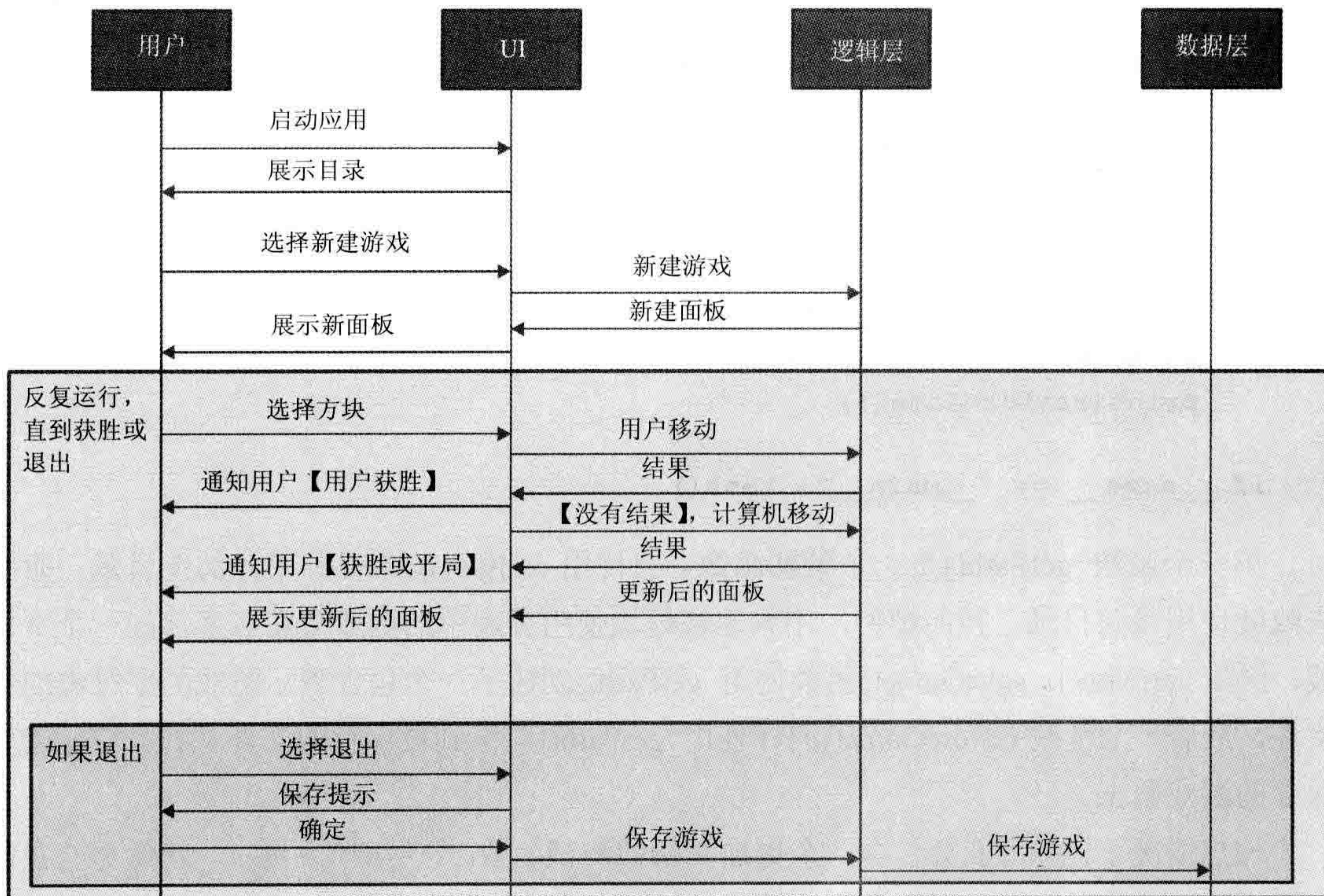
图 4-1 模块交互序列图
