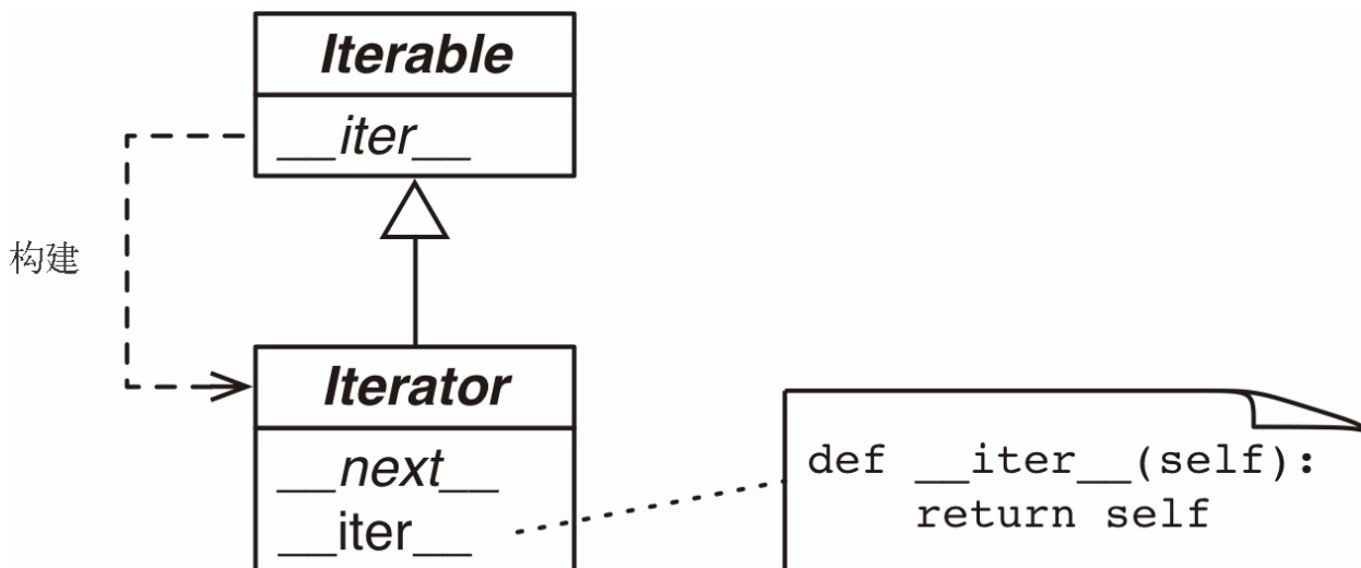
图 14-1: Iterable 和 Iterator 抽象基类。以斜体显示的是抽象方法。具体的 Iterable.__iter__ 方法应该返回一个 Iterator 实例。具体的 Iterator 类必须实现 __next__ 方法。 Iterator.__iter__ 方法直接返回实例本身
