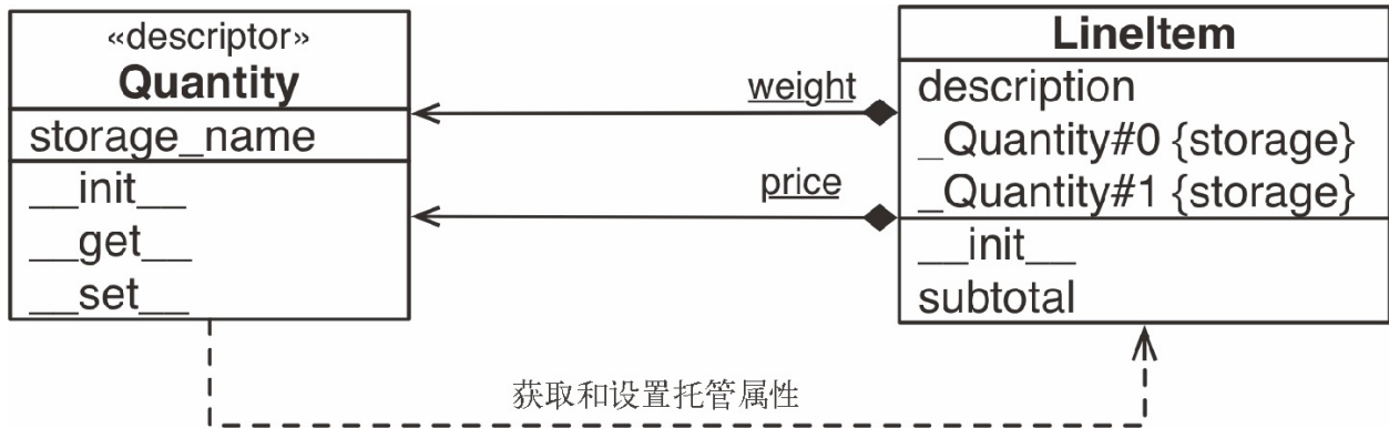
图 20-4: 示例 20-2 的 UML 类图。现在, Quantity 类既有 __get__ 方法, 也有 __set__ 方法; LineItem 实例中储存属性的名称是生成的, _Quantity#0 和 _Quantity#1
