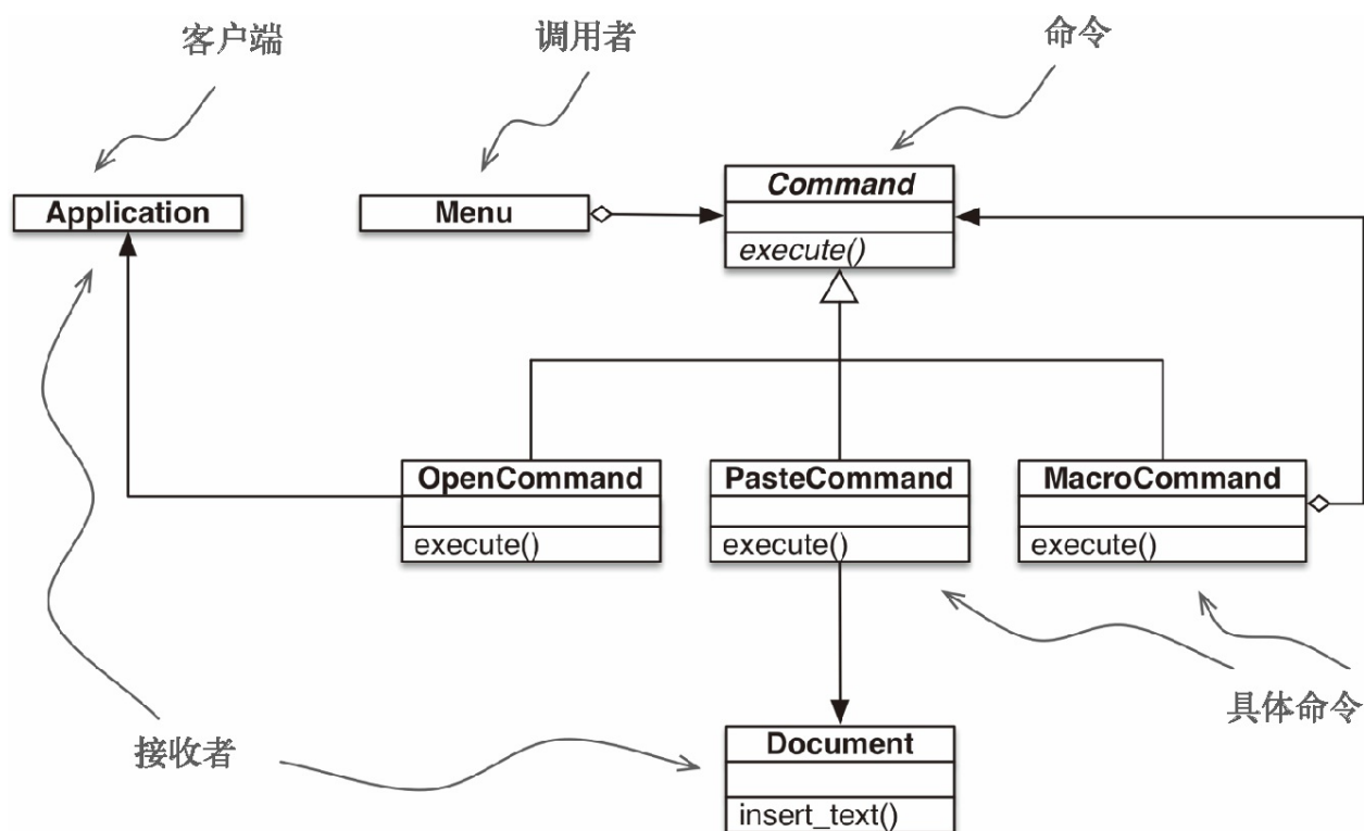
图 6-2: 菜单驱动文本编辑器的 UML 类图, 使用“命令”设计模式实现。各个命令可以有不同的接收者(实现操作的对象)。对 PasteCommand 来说, 接收者是 Document 。对 OpenCommand 来说, 接收者是应用程序
