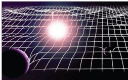
如果地球消失，周围时空就会开始震动，引力像涟漪一样传播
