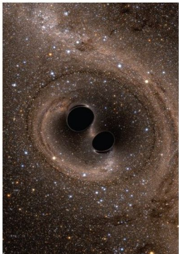
电脑模拟两个黑洞的碰撞
