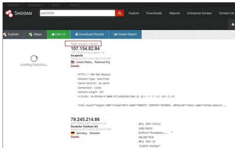
利用TCP9100端口,可轻松扫描出数万台各国的活动打印机
