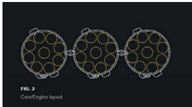
重型猎鹰并联了三组八角、九核心“梅林-1D”引擎
