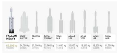
近地轨道(LEO)运载能力比较,最右为我国的“长征三乙”型运载火箭
