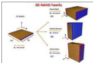
3D 闪存结构
