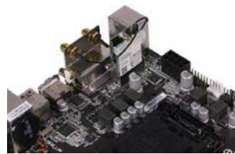
主板的供电设计升级到了5相
