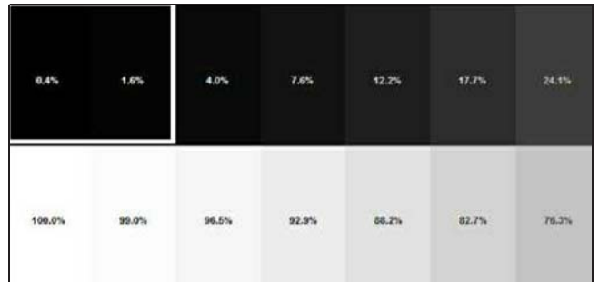
在对比度测试上Y700勉强能看清4%亮度和1.6%亮度的差别,在本次测试中属中游水准
