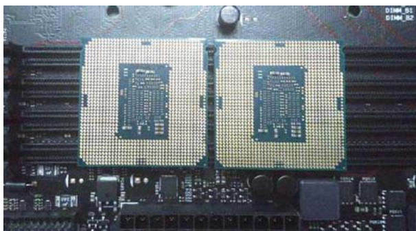
至强E3-1230V5(左)与Core i7 6700K(右)对比
