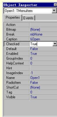
图 3-23 设置菜单的复选标志
