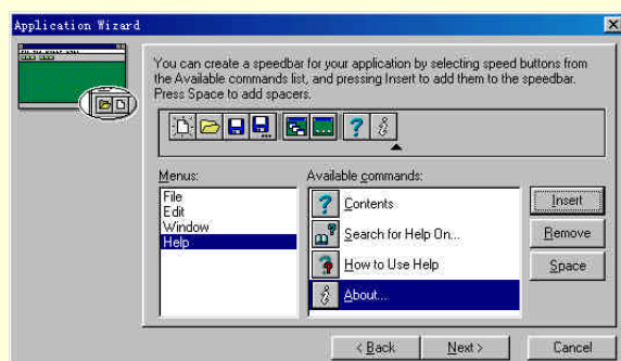
图 1-13 设计工具栏上的加速按钮
