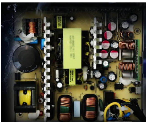
通过了 80PLUS 认证的电源品质更有保证
