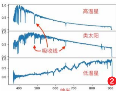
光谱来自郭守敬望远镜(LAMOST dr6)
