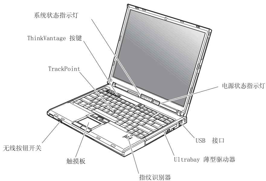
前视图
