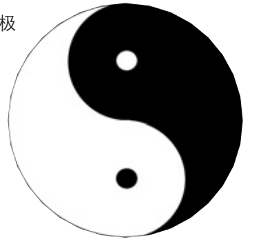
阴阳太极图
