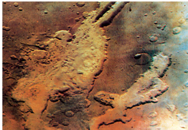
水手谷横跨火星赤道。
