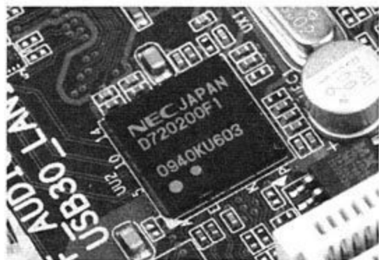
NEC D720200F1控制芯片让USB3.0接口的数据带宽提升至5Gbps
