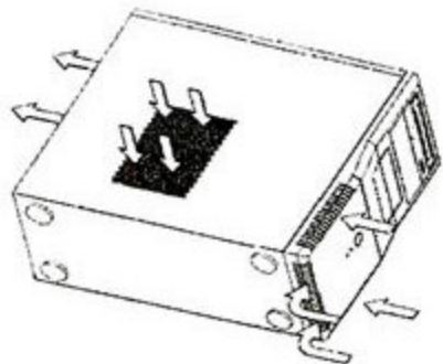
TAC 2.0规范的进风口示意图
