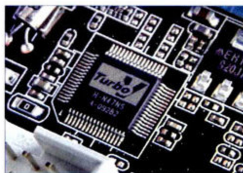
Turbo V O.C.芯片让华硕P55主板实现实时自动超频
