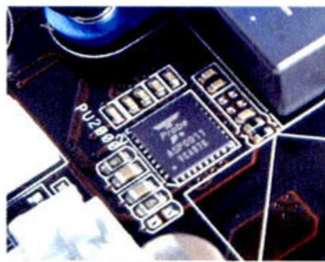
T.Probe芯片集侦测、调整、优化等功能于一体
