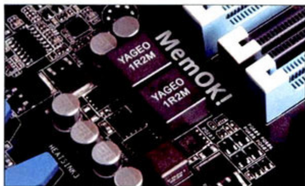
独立的两相供电电路, 为主板芯片组高效供电
