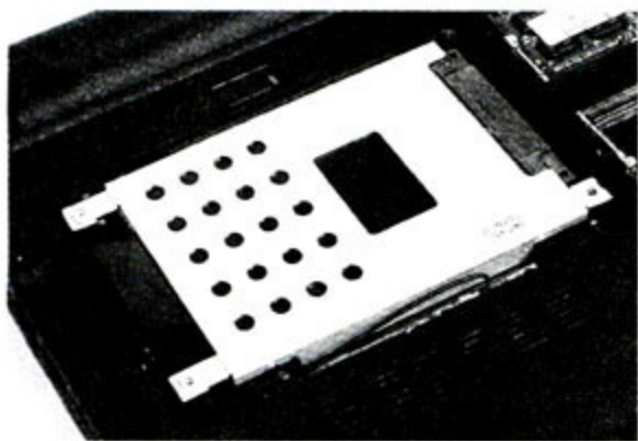
可拆卸的后盖设计让用户未来升级内存和硬盘时操作十分容易
