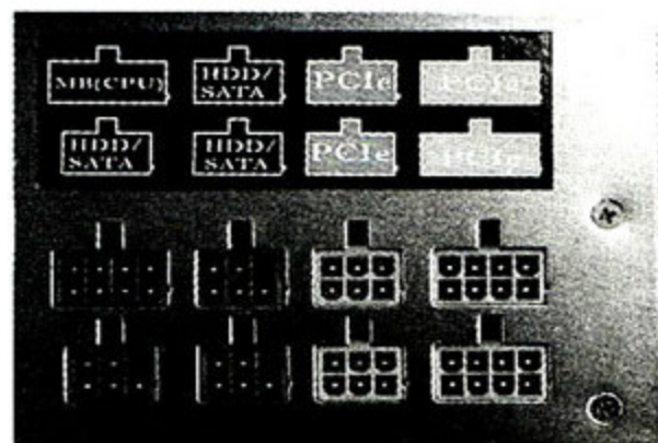
X7电源采用了模块式可拔插输出设计
