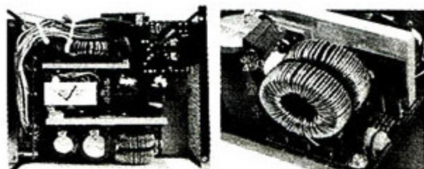
X7电源内部结构一览 交错式PFC拥有两个体积巨大的电感线圈
