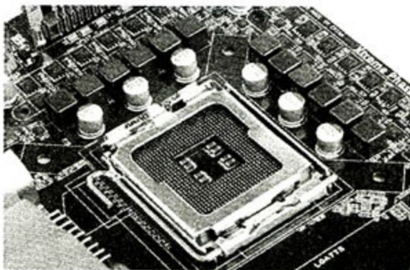
Extreme Design系列中的主流产品——P5P43TD PRO也采用12相供电设计
