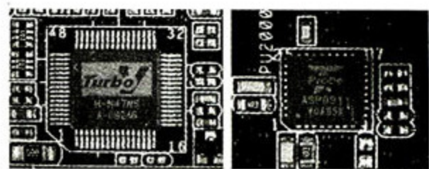
Turbo V在Turbo V EVO超频芯片和T.Probe监控芯片的帮助下实现实时超频
