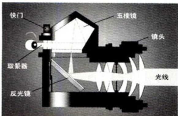
单反相机取景原理
