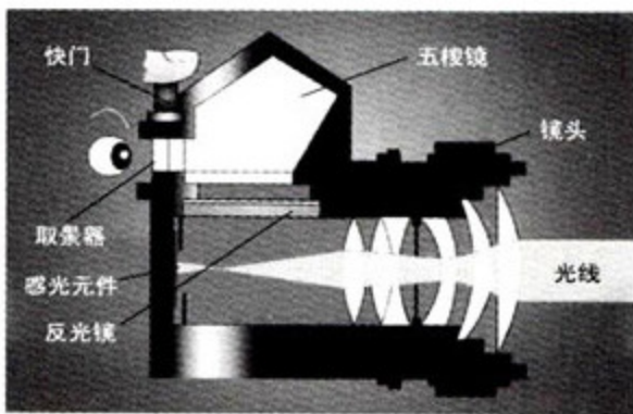
单反相机成像原理
