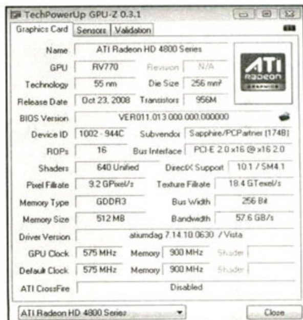
用GPU-Z可以看出蓝宝石Radeon HD4830白金版的显存频率并没有达到标称值
