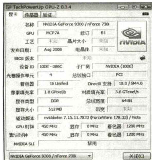
GeForce 9300硬件规格非常低,但却更实用
