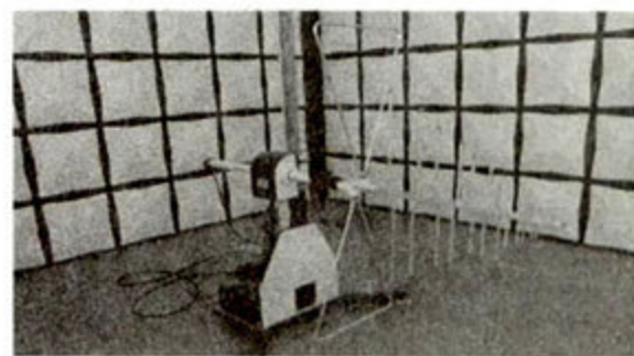
用于辐射测试的电磁辐射探测天线
