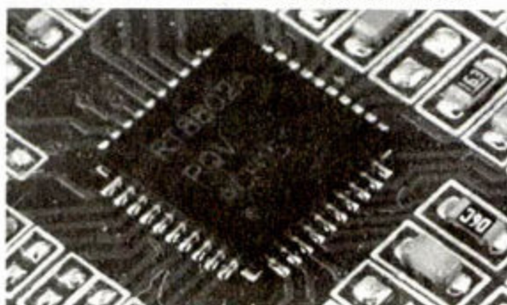
▼ RTCHEK RT8802A电压/频率控制芯片
