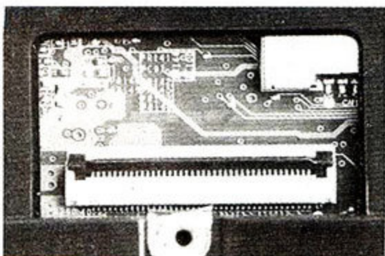
▲ SSD插槽的是供让SSD+HDD硬盘混搭成为可能
