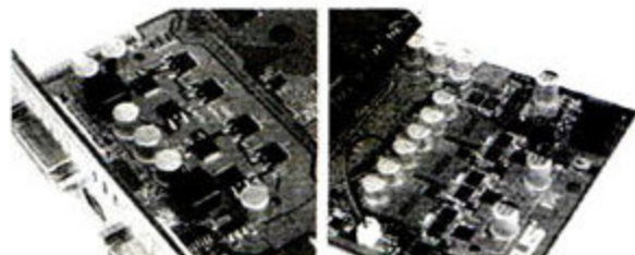
▲“游戏显卡专家”显卡采用2+1相供电设计,并且直接放在了接口旁边 ▲“巨狮”显卡采用3+1相供电设计,并且远离输出接口
