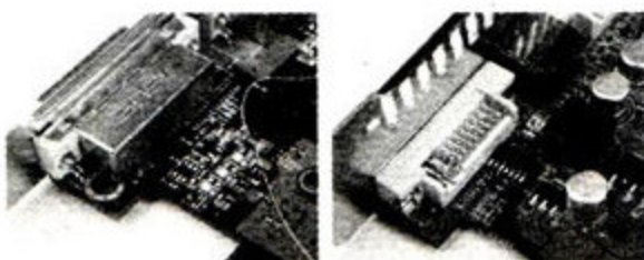
▲“巨狮”显卡的接口 ▲“游戏显卡专家”显卡加上了金属屏蔽网,且不仅没有金属屏蔽网,而且低通电路饱满且电磁干扰就在旁边
