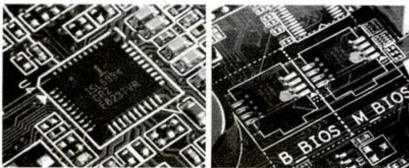
▲ 主板的Intersil ISL6334 PWM控制芯片
