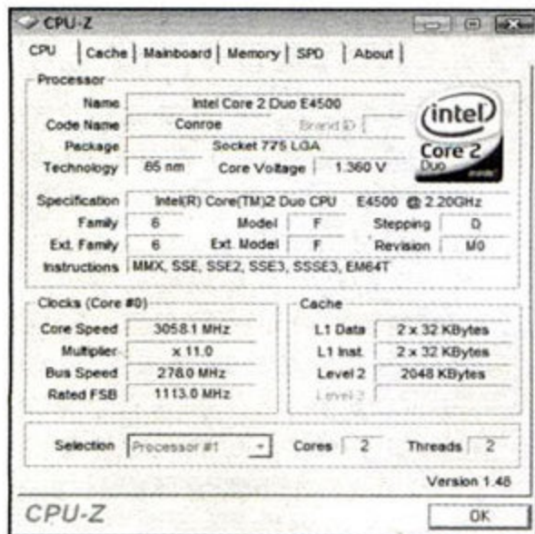
▲ 1.4V电压下E4500稳定超频至3.05GHz
