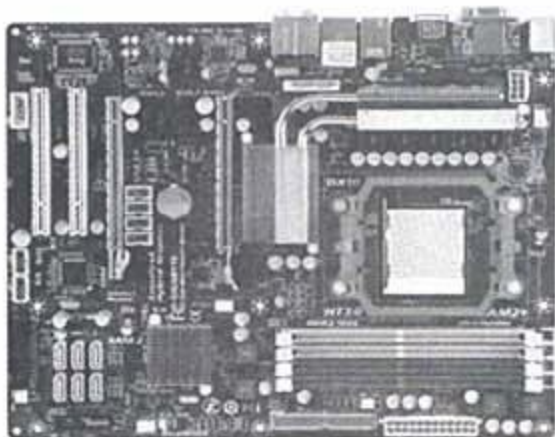
▲ 支持DX10整合显示核心的790GX主板。
