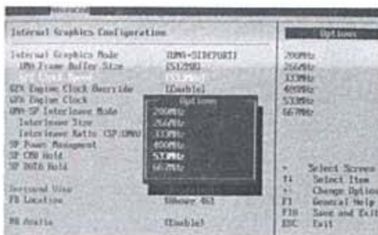
780G主板的显示核心频率调整。
