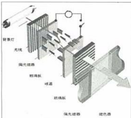
液晶成像原理
