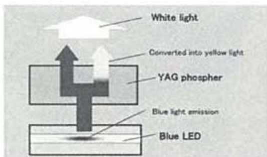
白光LED的发光原理
