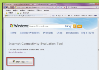
ICET 主界面
