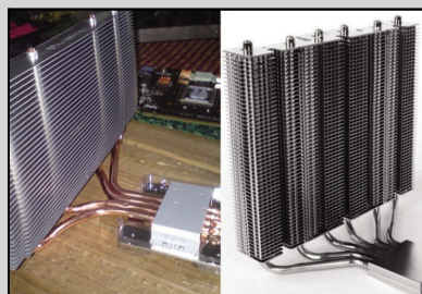
● 改造后的散热器和“喷火”对比
