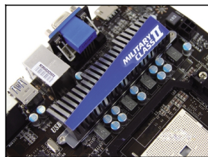
● SFC 电感 + 固态电容设计的供电部分
