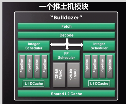
● 标准的推土机模块示意图
