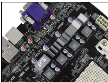
● 4 相的 CPU 供电系统中规中矩
