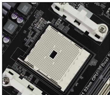
● FM1 处理器插座, 无法支持 AM3 处理器, 购买时切记
