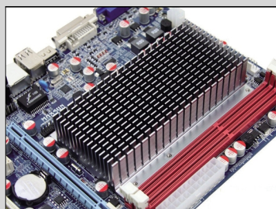
● 测试用的 APU 主板,仅依靠这个散热片散热
