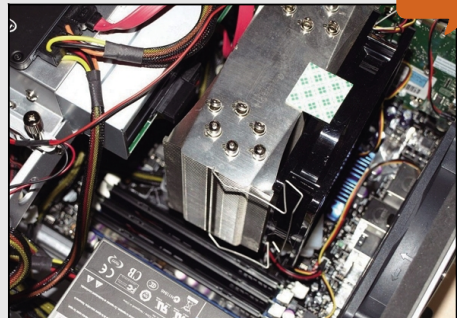
● 散热器螺丝没旋紧,歪向一边
