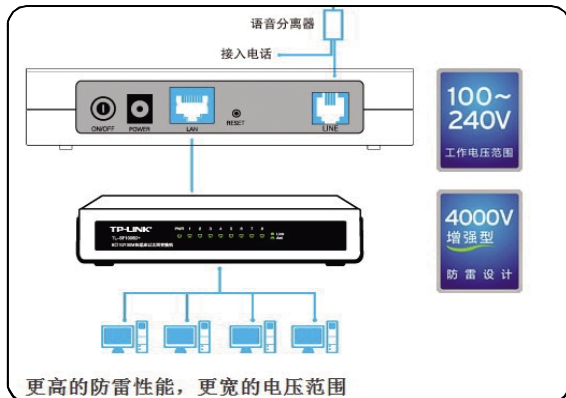
●防雷路由器具有一定程度的防雷作用
