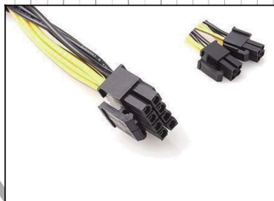
● 用于主板供电的 8 针魔术接口,可拆分为 4+4 针
