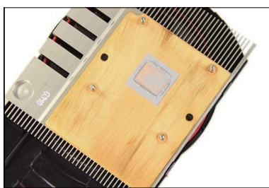
● 底部采用先进的均热板
