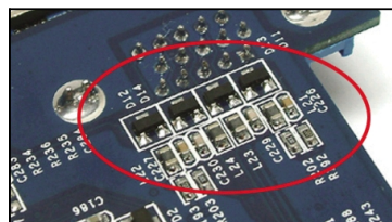
● 这些小贴片就是显卡低通滤波电路中非常重要的一部分
