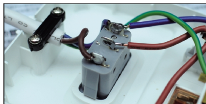
●开关焊接工艺优秀,还加了地线
