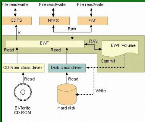
● EWF 的工作原理示意图
