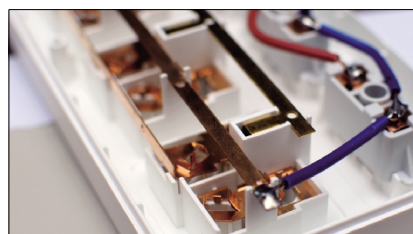
●采用一体式插套设计,导线更粗
