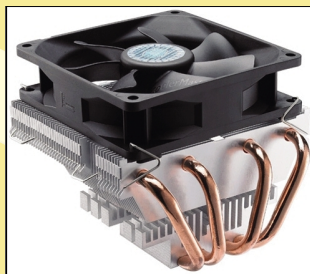
● 带热管的下压式散热器安装时要注意不要将热管朝向发热源
