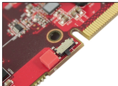
● 用户拨动这个小开关，就可实现超频
