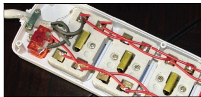
●普通插座导线细不安全
