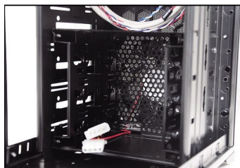
●硬盘和散热风扇采用一体式设计
