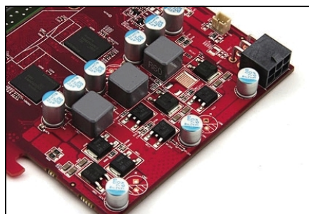
●HD6770 恒金 1G 采用分离式供电
