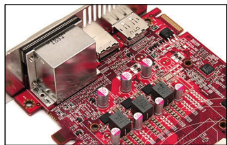
●分离式供电设计,避免了干扰现象
