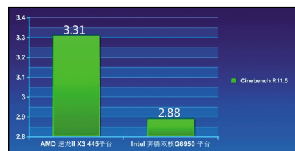
● Cinebench R11.5 测试结果
