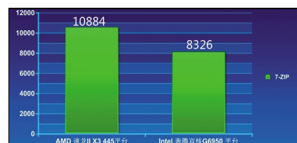
● 7-ZIP 测试结果
